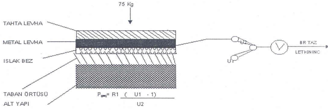
Şekil 20 – Zemin yalıtıklık direncinin ölçülmesi
