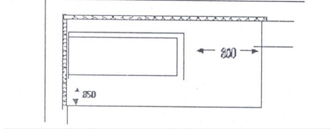
Şekil - 21 Banyoda koruma bölgesi
