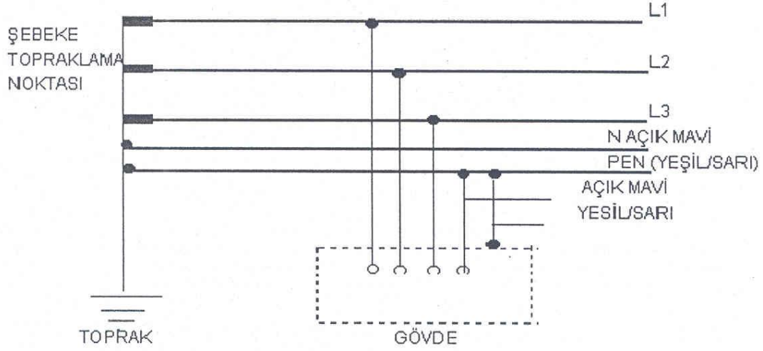
ŞEKİL 1-2 NÖTR VE KORUMA İLETKENLERİ AYRI ÇEKİLMİŞ TN SİSTEMİ (TN-S)
