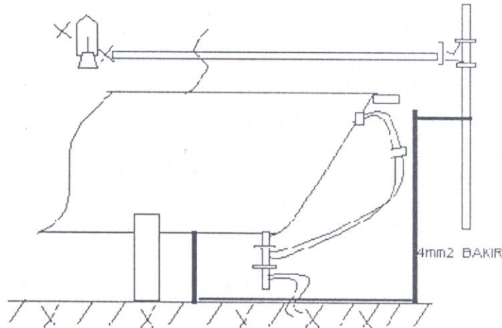
Şekil -22 Potansiyel dengelemesinin yapılışı
